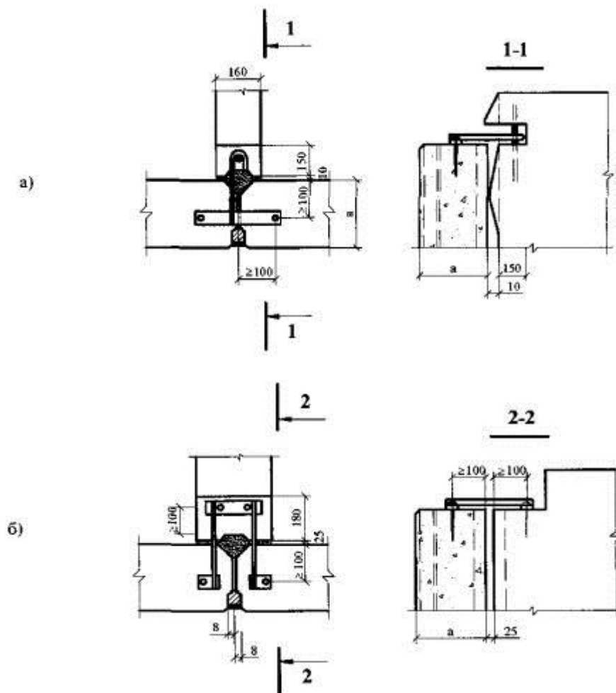
а) узел соединения; б) узел крепления к ячеистобетонной поперечной стене.
