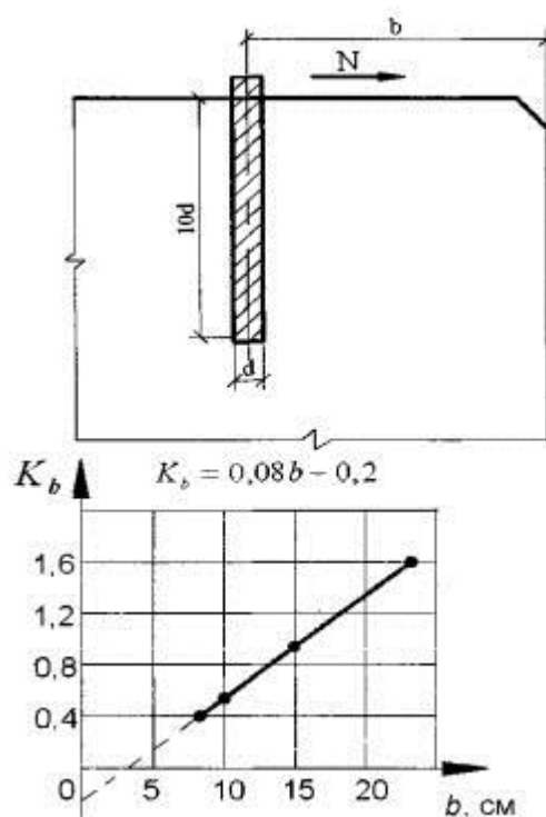
Рисунок 3.2 - График зависимости между несущей способностью забивного или вклеенного анкерного крепления и расстоянием «b» от грани панели
