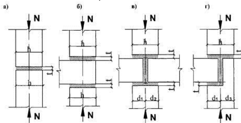
а - стык контактный; б - одностороннее платформенное опирание с перекрытием, заведенным на всю толщину стены; в - стык платформенный; г -стык с комбинированным опиранием
